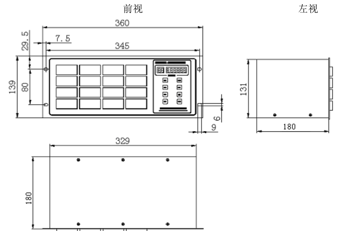
FYXH-16.A1 外形尺寸图
